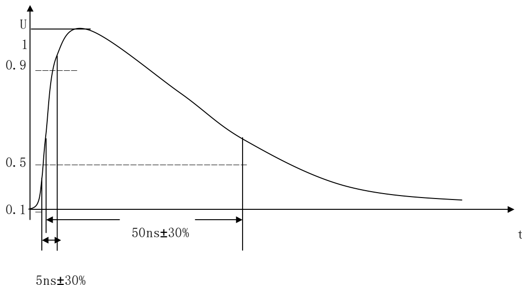
图 3 50Ω负载时单脉冲波形
